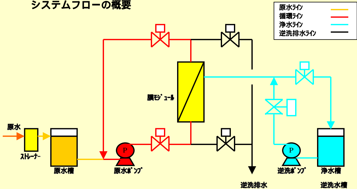
〈 基本 フ ロ - 図 〉
